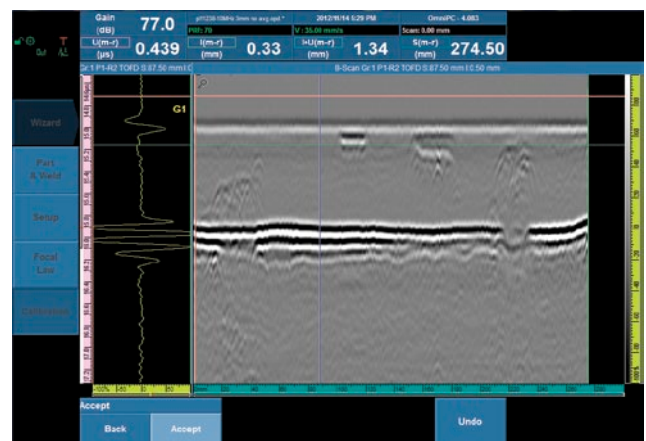
经过直通波拉直操作后的TOFD数据
